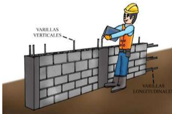
Figura 55: Pared estructural de mampostería reforzada
