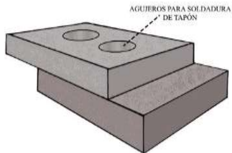
Figura 118: Soldadura de tapón
