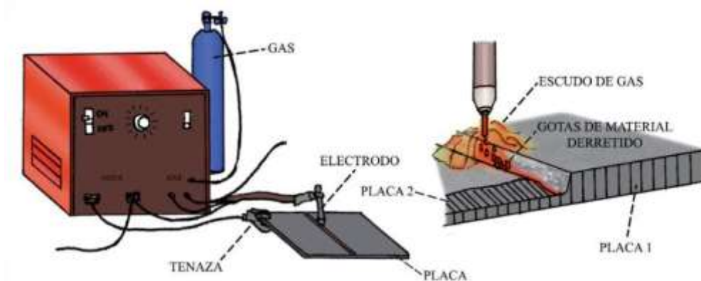
Figura 111: Suelda tipo GMAW
