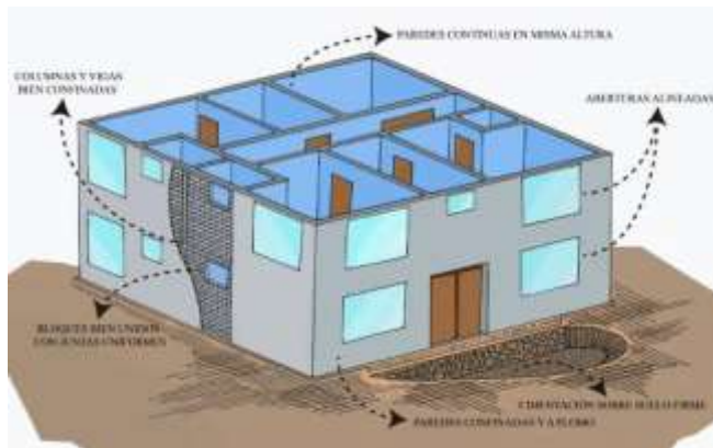
Figura 10: Una buena vivienda sismo-resistente
