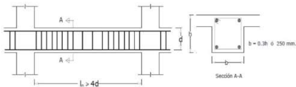
Figura 87: Características de la sección de las vigas
