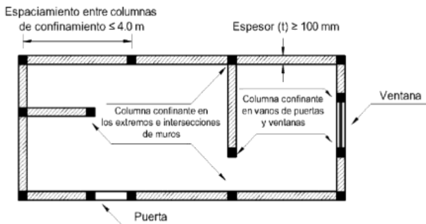
Figura 73: Ubicación de columnas confinantes
