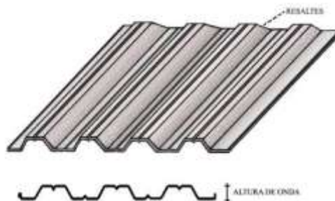
Figura 109: Steel deck para losas, cubiertas
