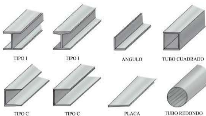
Figura 103: Algunos tipos de perfiles estructurales que se encuentra en el mercado
