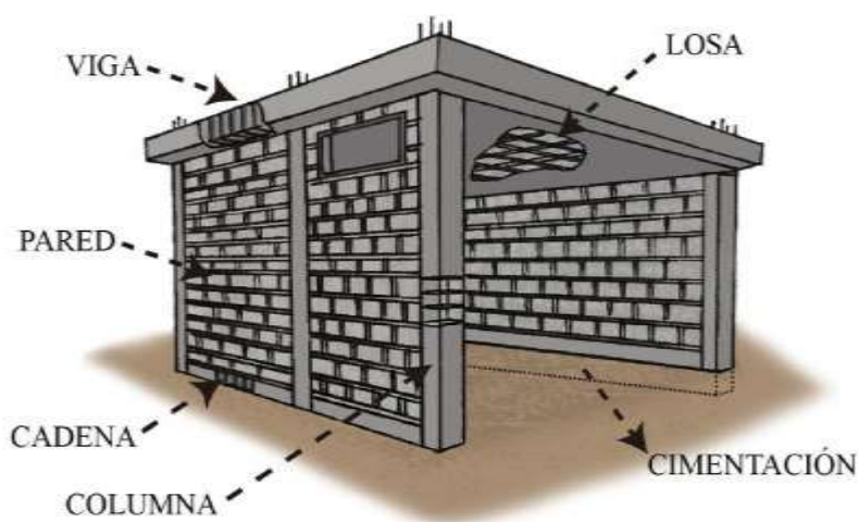
Figura 5: Elementos estructurales que conforman una vivienda
