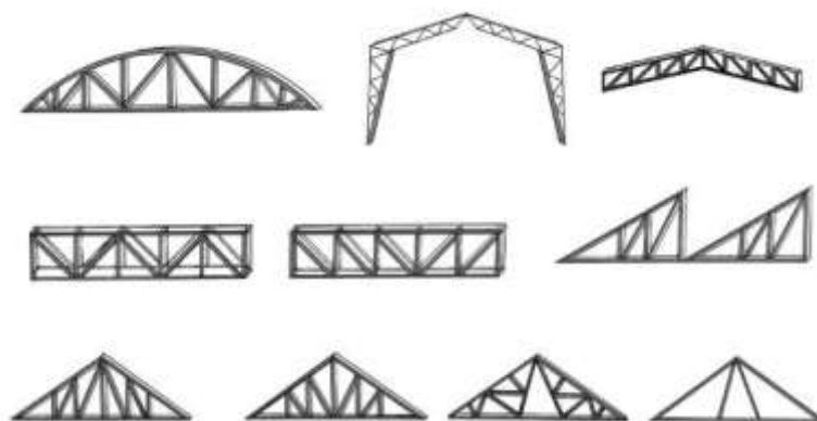
Figura 108: Tipos de cerchas
